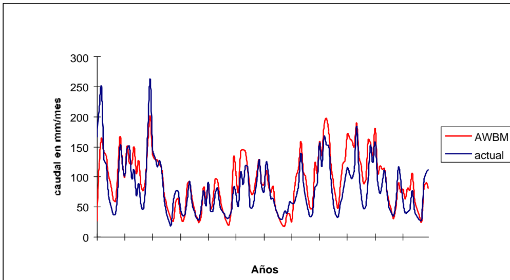
Figura 2.8 Comparación del caudal real y el simulado. Río Ovejas, AWBM
