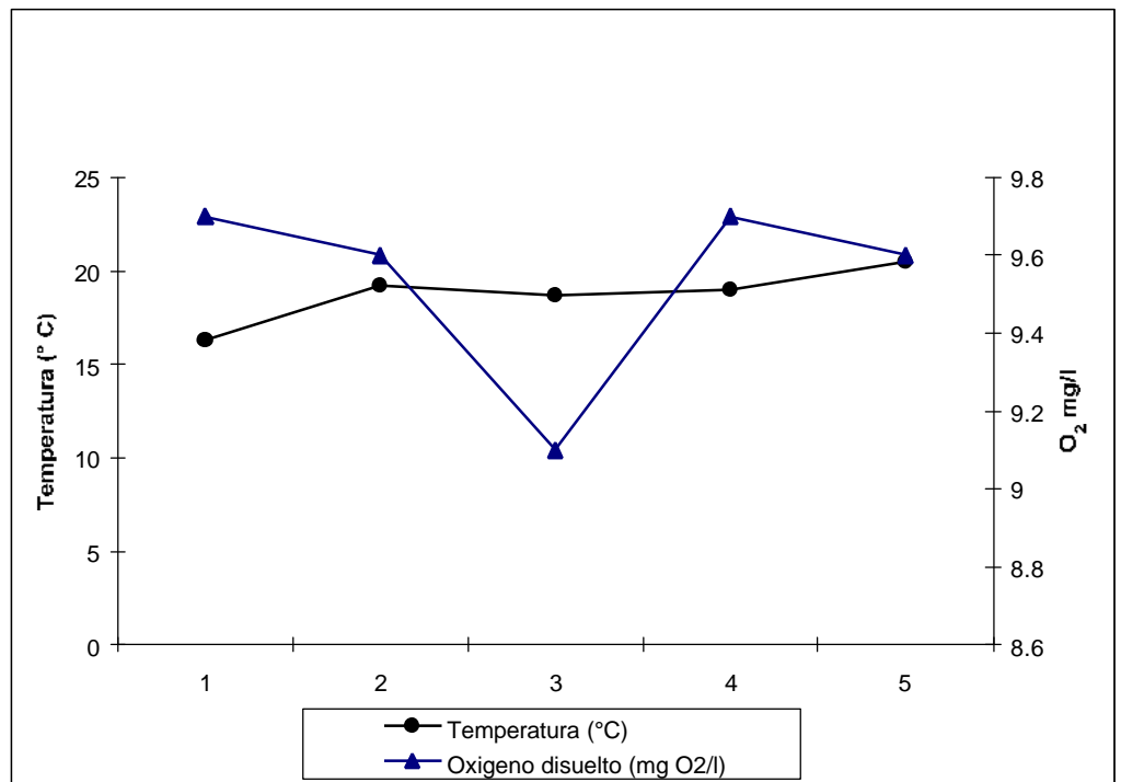
Figura 3.6 Evolución de la temperatura y del oxígeno disuelto entre las estaciones
