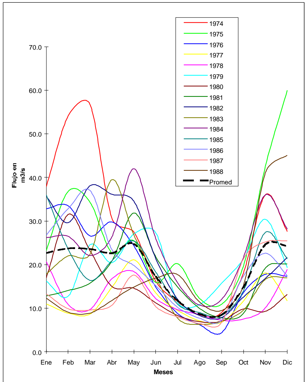
Figura 2.2 Variación de Flujo del Río Ovejas en m 3 /s de 1974-1988
