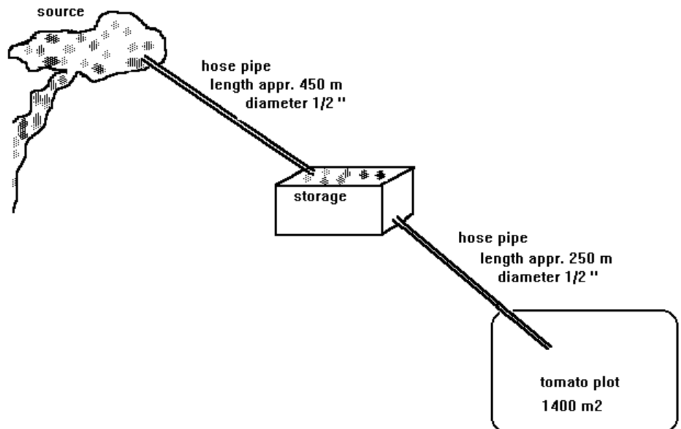
Figura 3.2 Técnica local de riego aprovechando la gravedad
