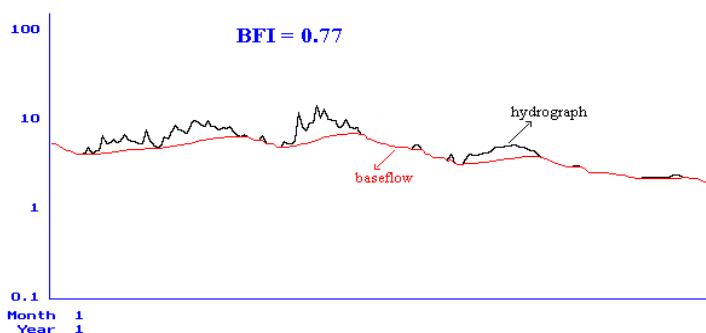
Figura 2.6 Programa AWBM de Balance Hídrico. Determinación del Índice de Caudal Base; BFI
