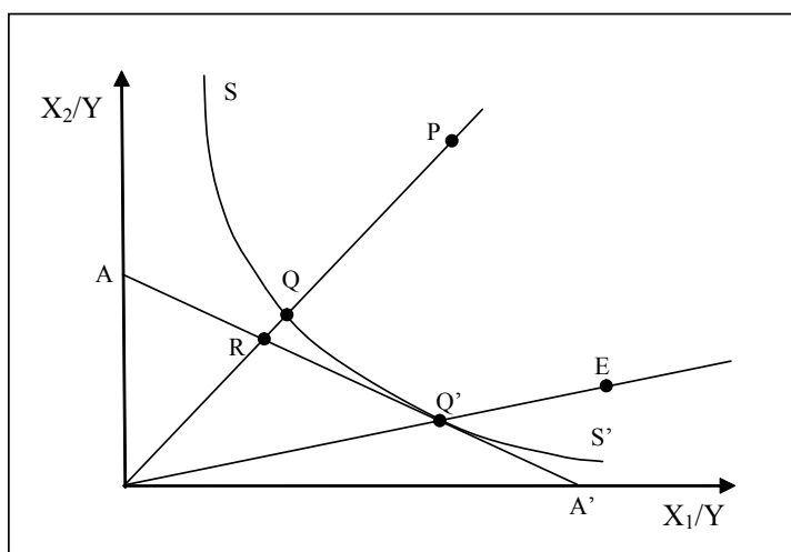
Figure 1. Représentation graphique (Farrell 1957) de l'efficacité technique et de l'efficacité allocative.
